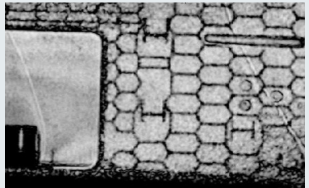
Airbag-Abdeckung: Materialdichteschwankungen und Defekte im Bauteilinneren nachweisbar.
